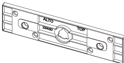
n° 1 base de montagem mounting base
