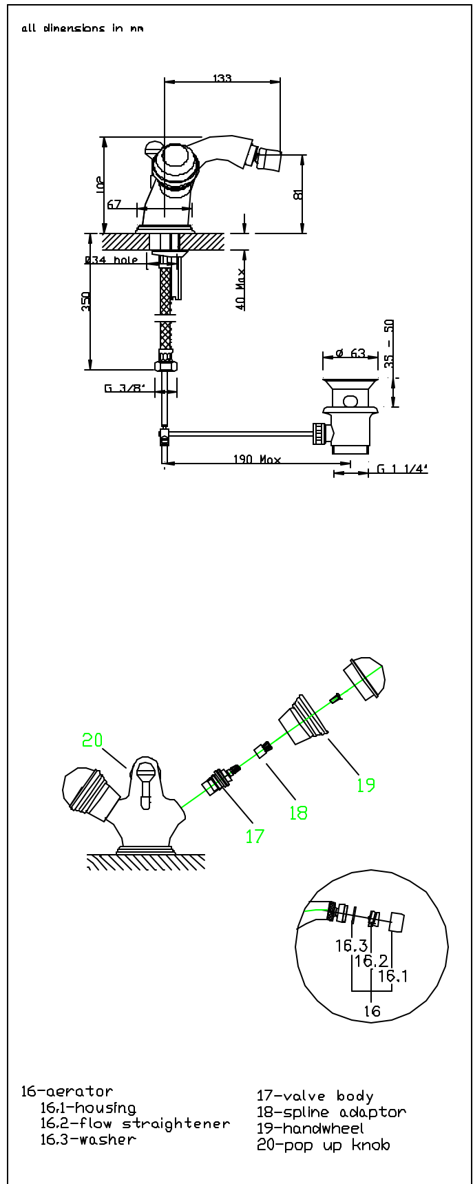
King monobloc bidet mixer
